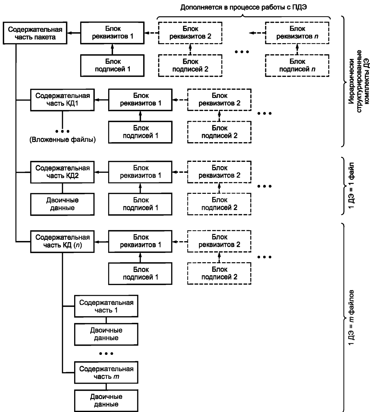
Рисунок В.1 — Логическая структура ПДЭ
